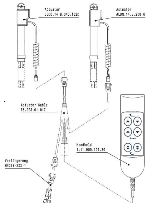
Elektrischer Antrieb mit Kabelsatz und Handheld
